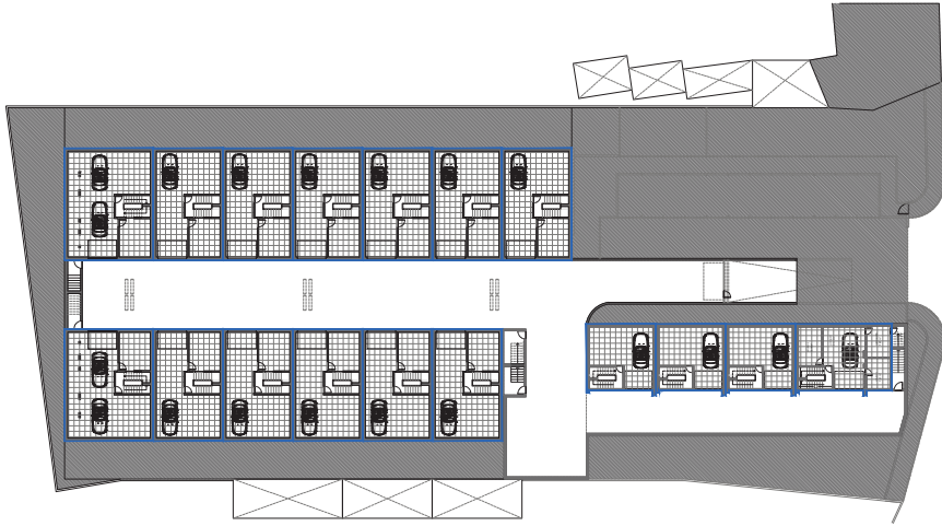
Planta piso -1
