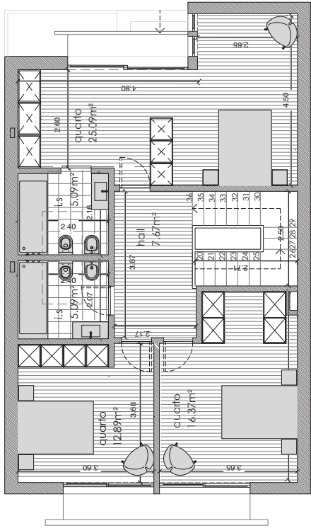
Planta Piso 1_ tipologia 1 98.31 m²
