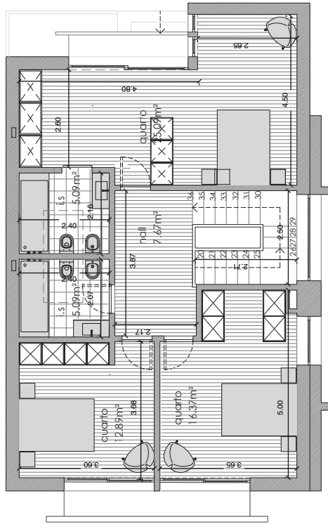
Planta Piso 1_ tipologia 2
