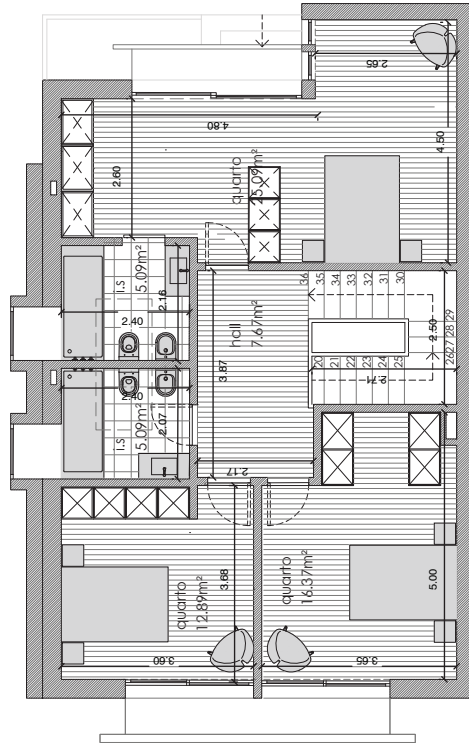
Planta Piso 1_ tipologia 3
